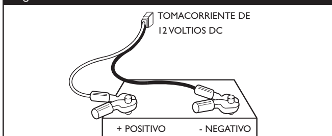
Figura 40 — Conexiones de la Batería
